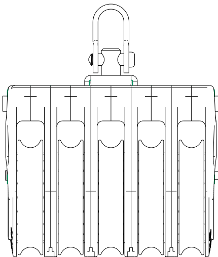
SCALE 1:2
